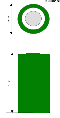
CEI C cellule seule
